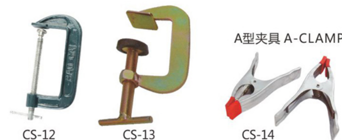
G型夹具 G-clamp 使用范围/Available usage: 50/ 75/ 100/ 125/ 150 mm
