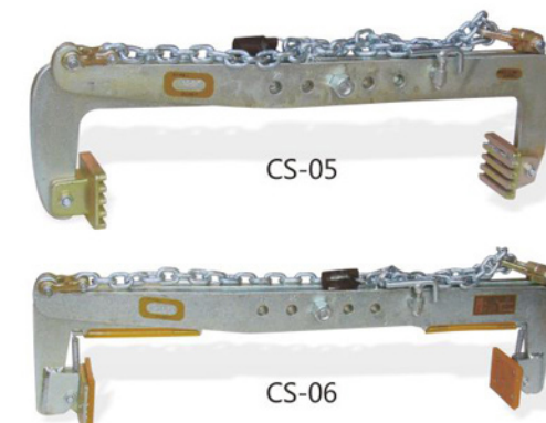
F型石材专用夹具 F-Model slab clamp 使用范围/Available usage: 180-1250mm 最大负荷/Max loading: 300-1500kg
